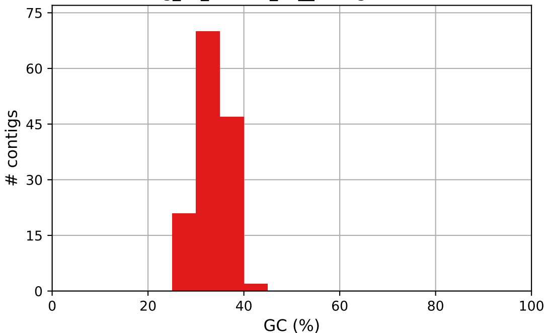
velvetg_on_dataset_98__Contigs GC content
